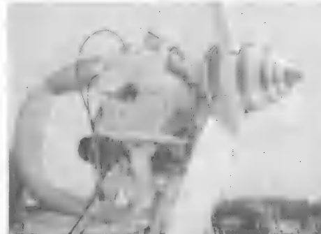
Силовая установка мотопланира «Гусь-1» с двигателем АП-17.
